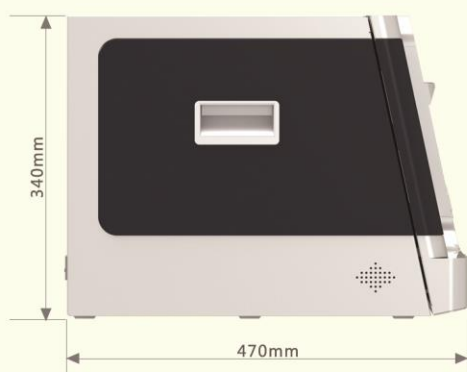
侧视图 ▲
