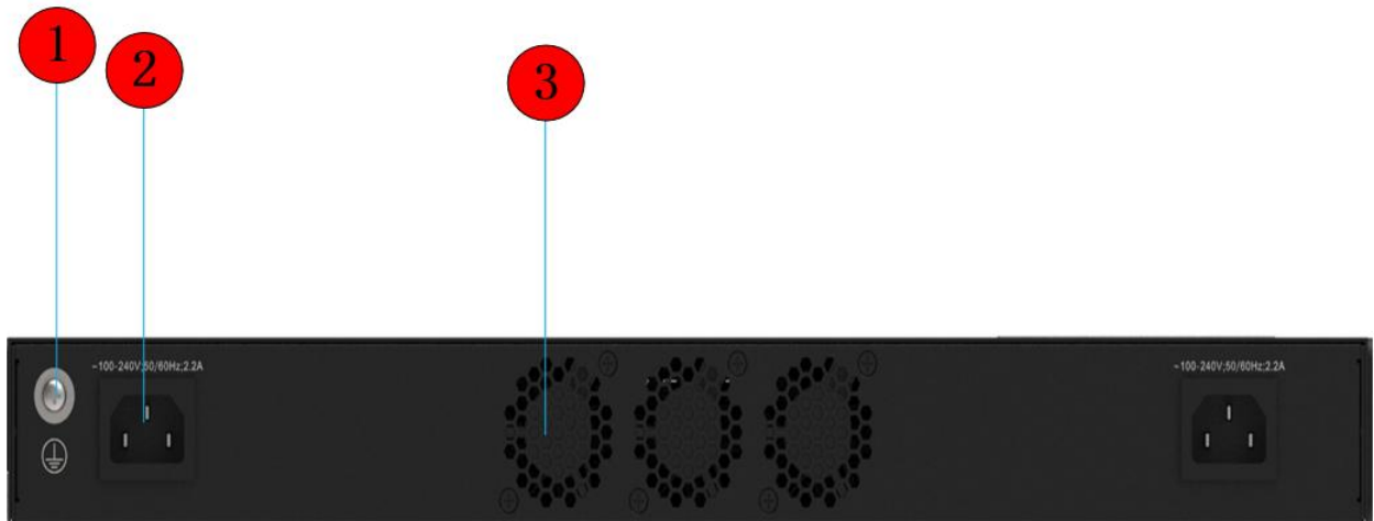
图 1-15 S6220E-48S4X-D 后面板示意图
