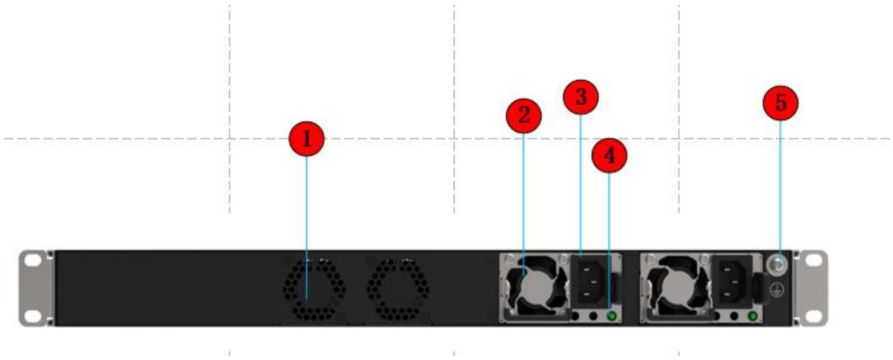
图 1-13 S6220E-48T4X-P 后面板示意图
