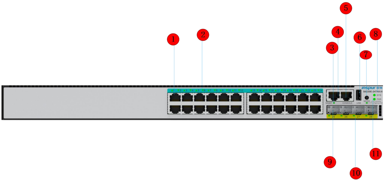
图 1-4 S6220E-24T4X-P 前面板示意图
