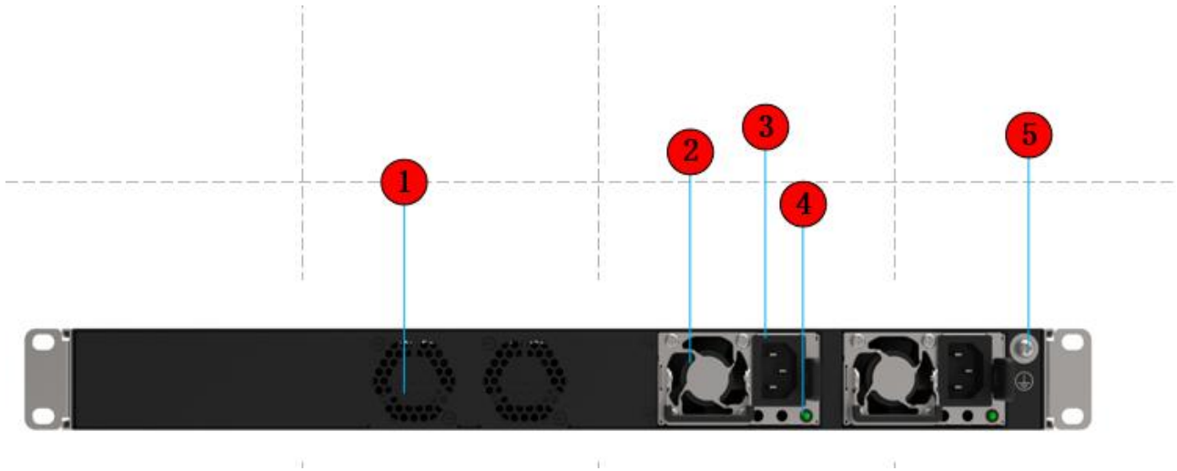
图 1-11 S6220E-48T4X-P 后面板示意图
