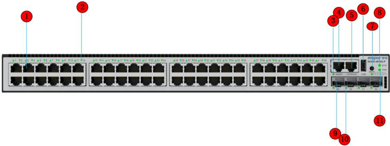
图 1-1 S6220E-48T4X-P 前面板示意图
