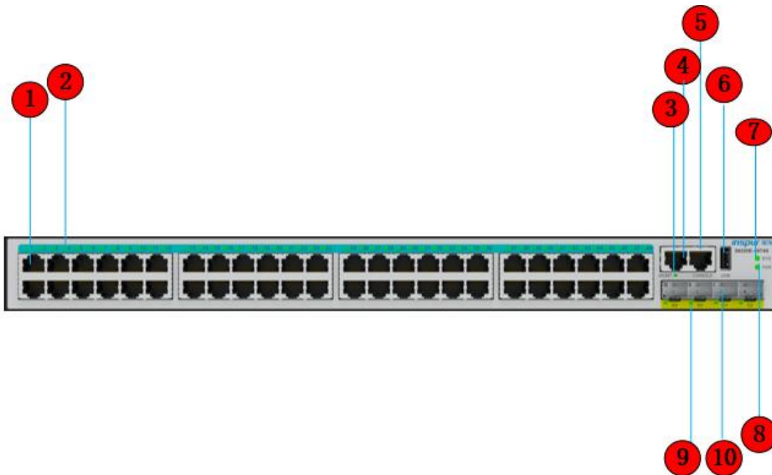
图 1-7 S6220E-48T4X 前面板示意图
