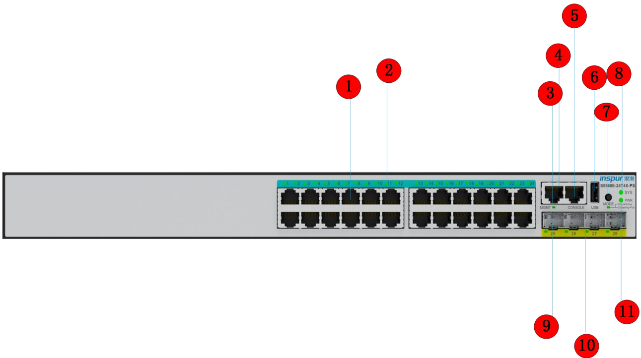
图 1-10 S5560E-24T4S-PS 前面板示意图
