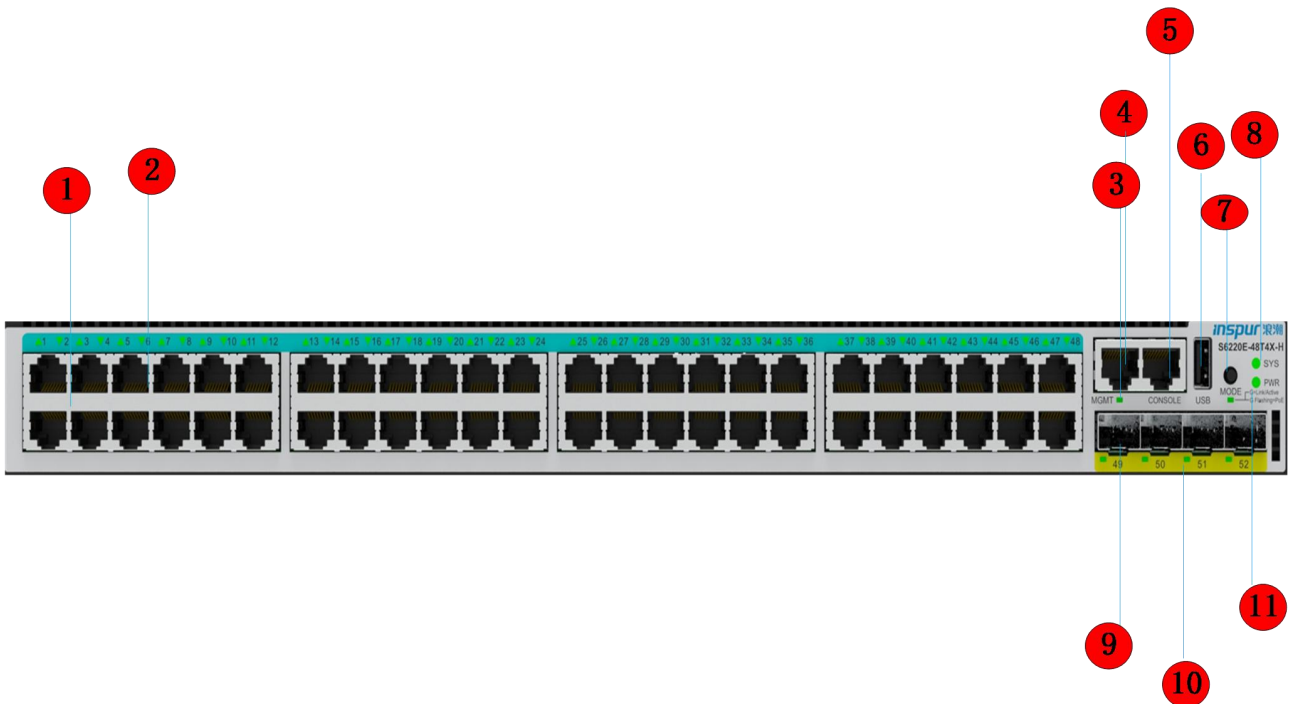
图 1-3 S6220E-48T4X-H 前面板示意图
