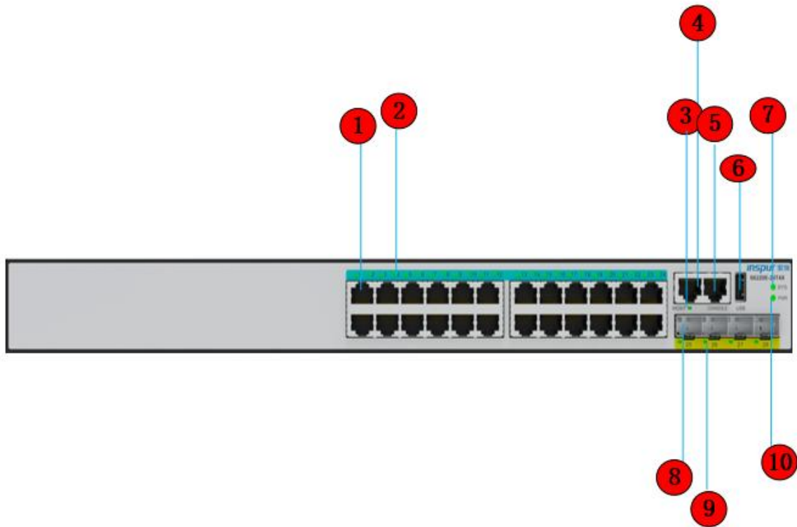
图 1-6 S6220E-24T4X 前面板示意图
