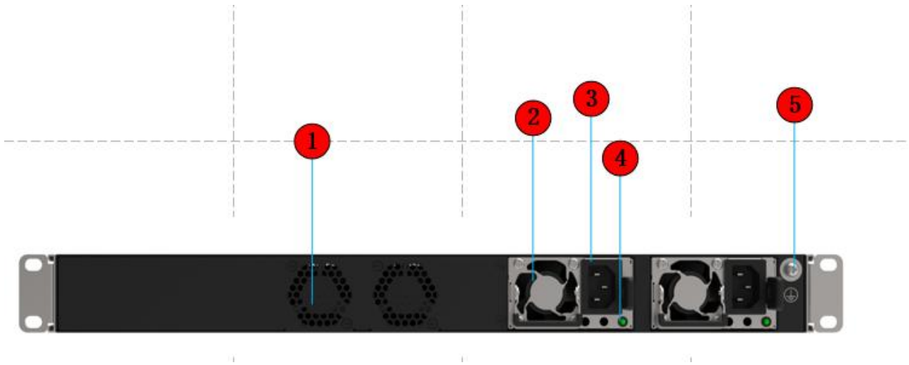
图 1-14 S6220E-48T4X-P 后面板示意图
