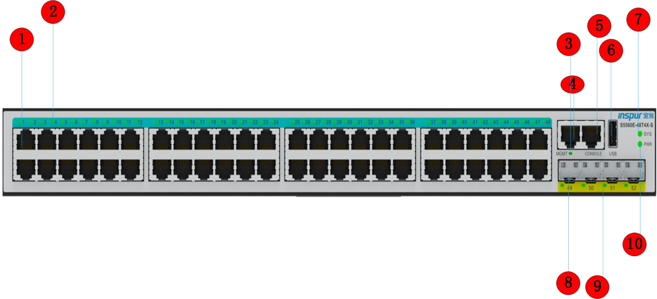
图 1-9 S5560E-48T4X-S 前面板示意图
