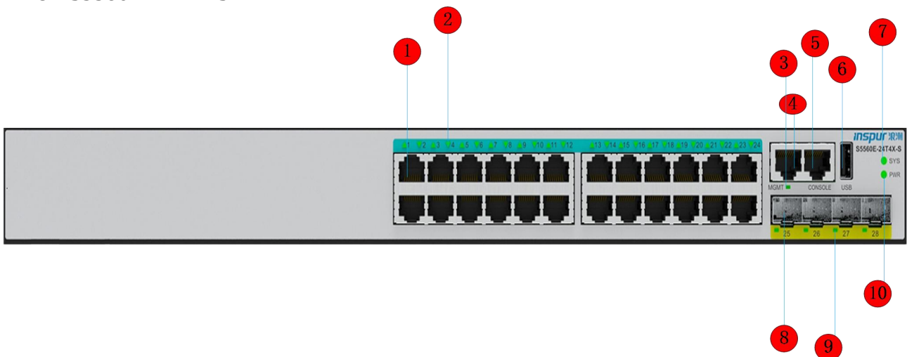
图 1-8 S5560E-24T4X-S 前面板示意图
