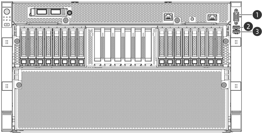
图 5-4 前面板接口（示例：16 盘配置）
