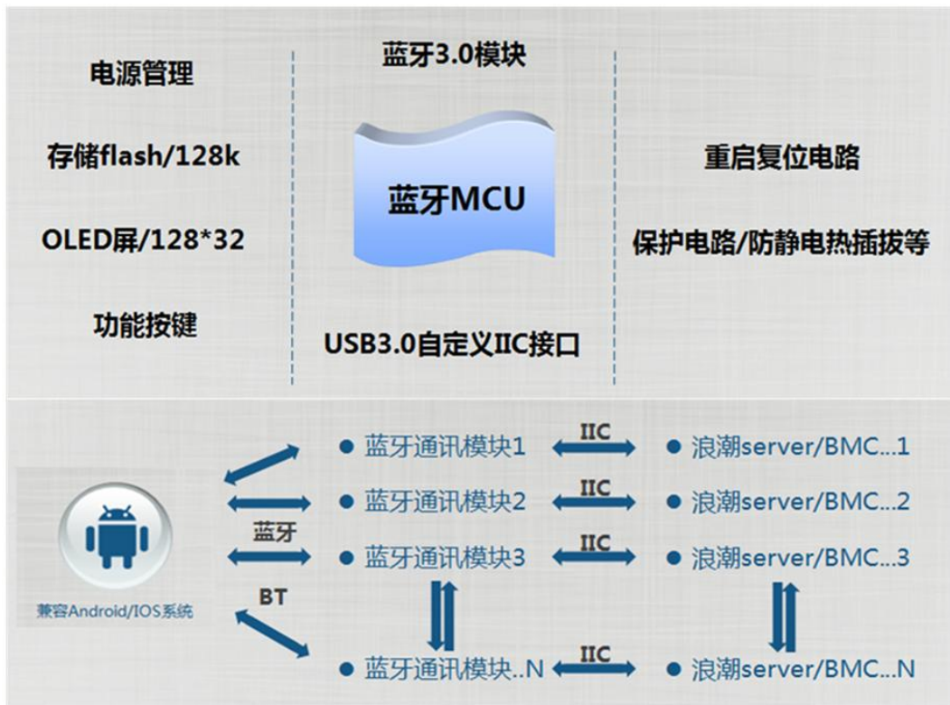
图 5-20 LCD 子系统工作原理
