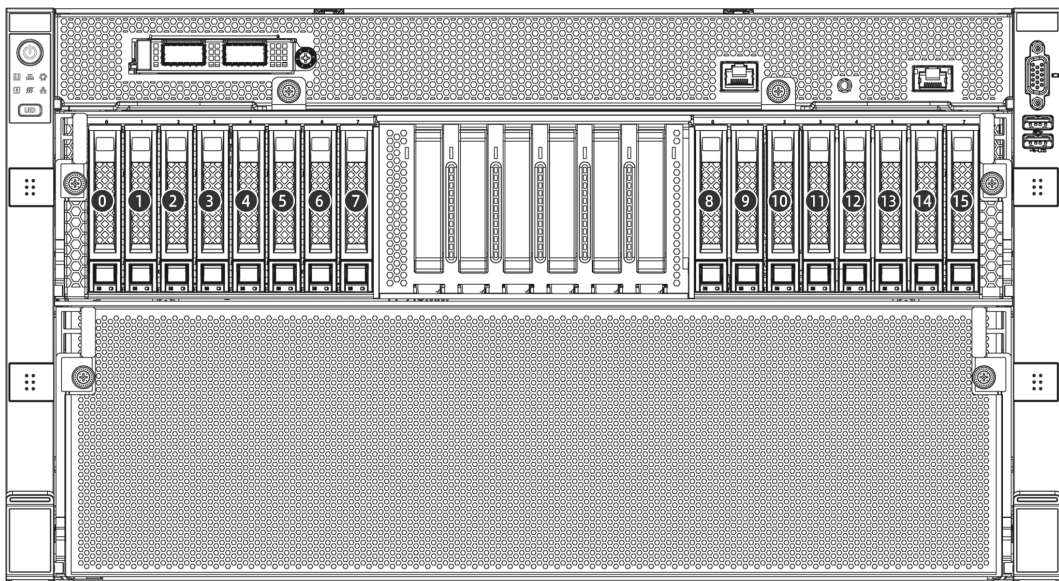
图 5-12 硬盘编号
