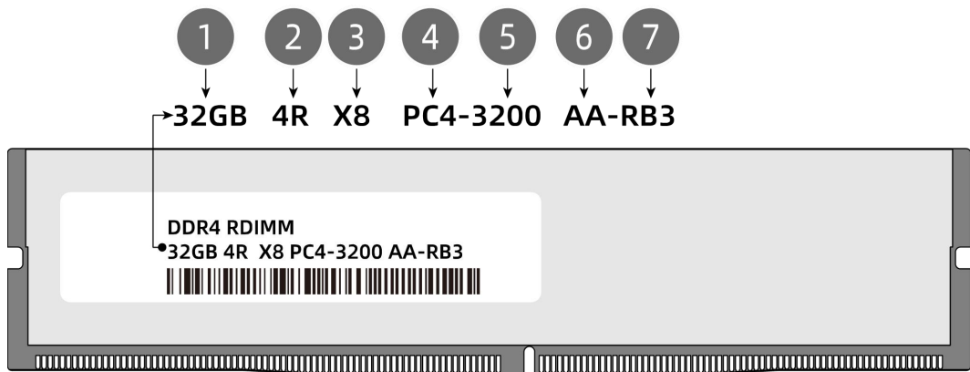
图 5-8 内存标识
