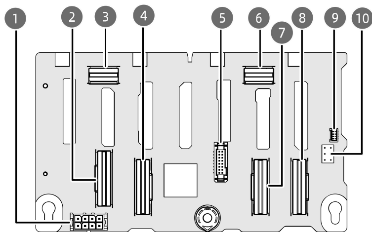
图 5-23 8 × 2.5 英寸硬盘 (8 × SAS/SATA/NVMe) 背板
