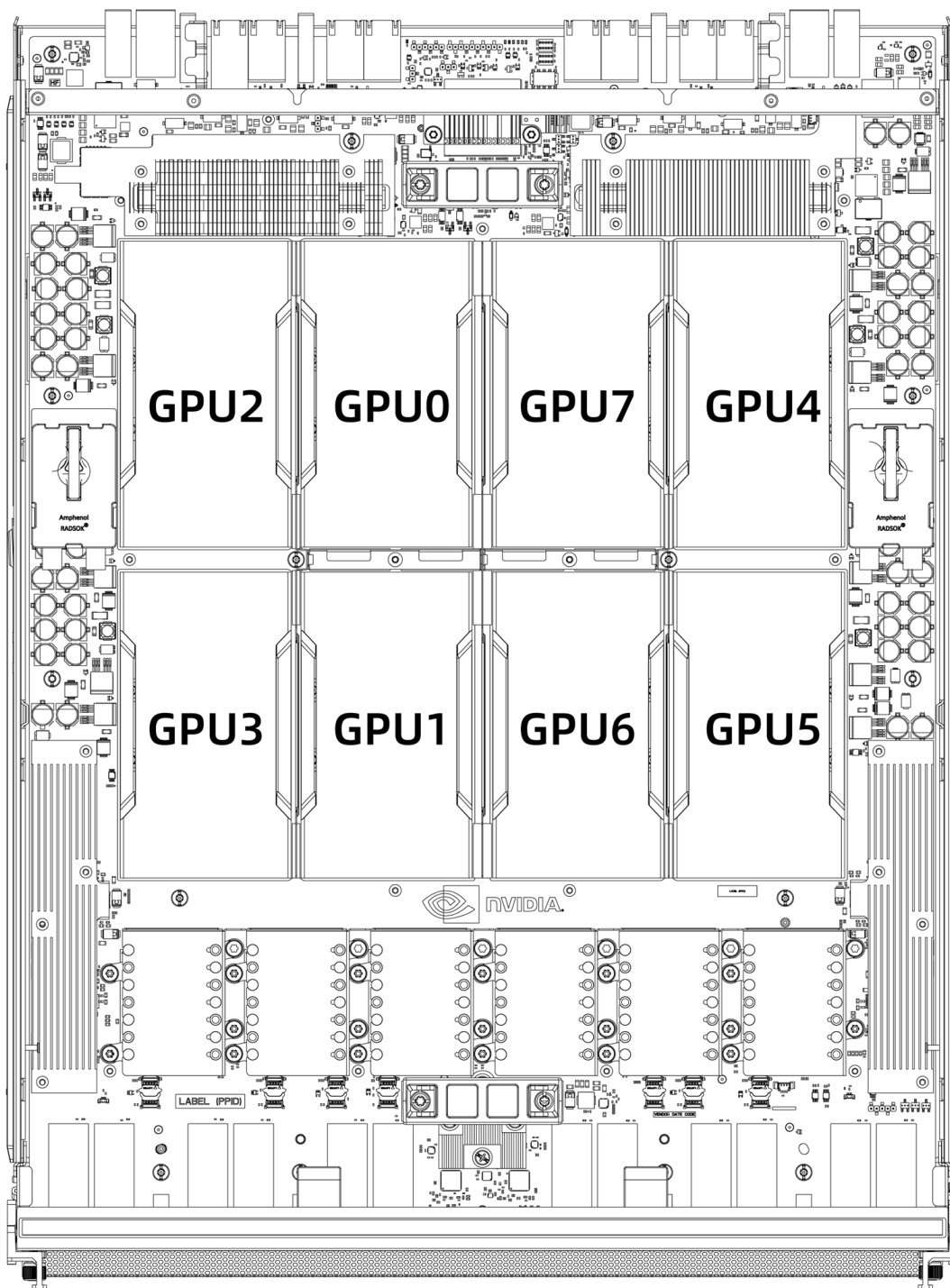
图 5-24 GPU 模组 GPU0-GPU7 顺序示意图
