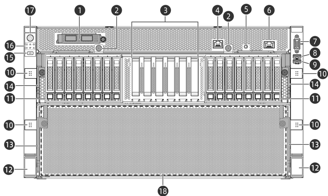
图 5-1 前面板外观
