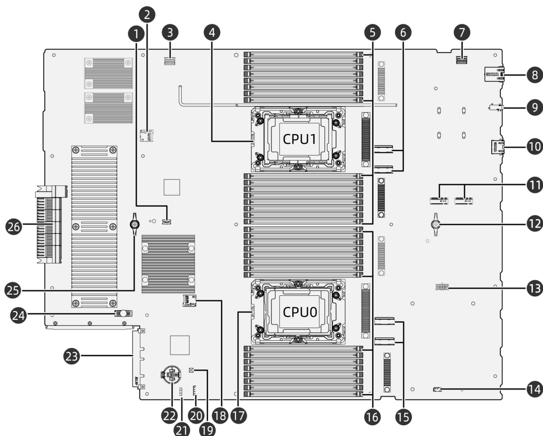
图 5-22 主板
