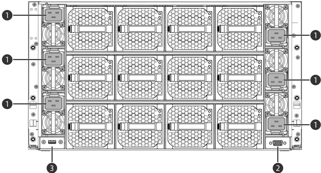
图 5-7 后面板接口（8 盘配置和 16 盘配置后面板接口设计一致）
