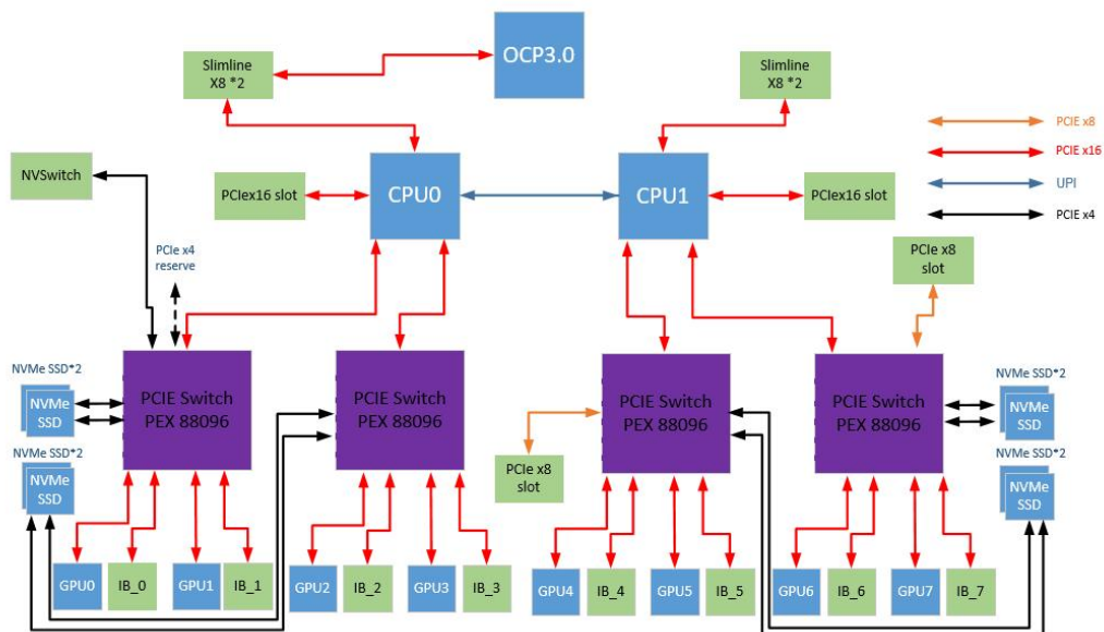
图 4-1 NF5688M6 逻辑结构 (8 盘配置)
