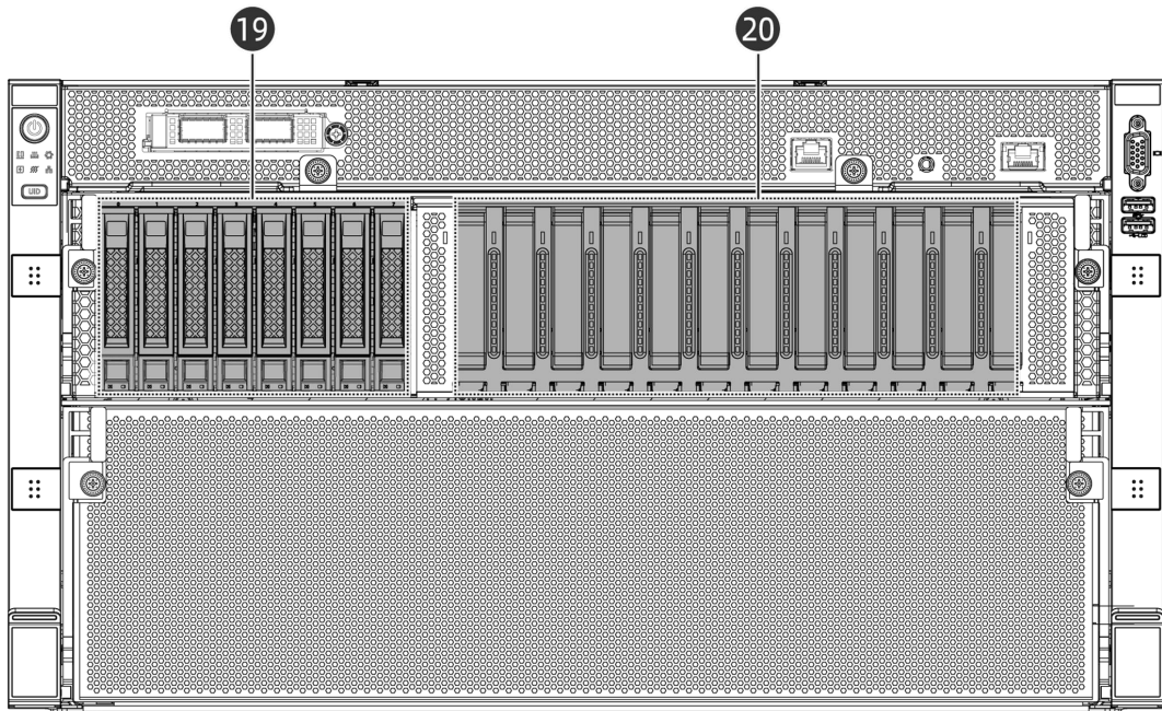
图 5-2 前面板外观
