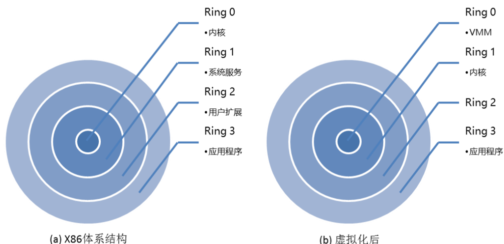
图 3.2.1-1 特权级
