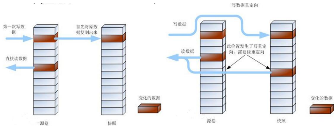
图 4.2.2-1 快照技术
