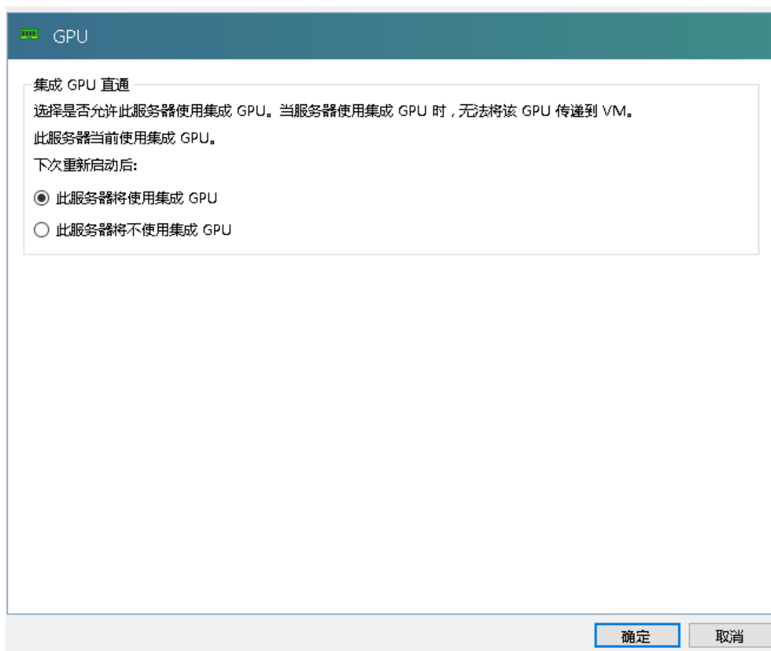
图 4.1.3-1 GPU 配置
