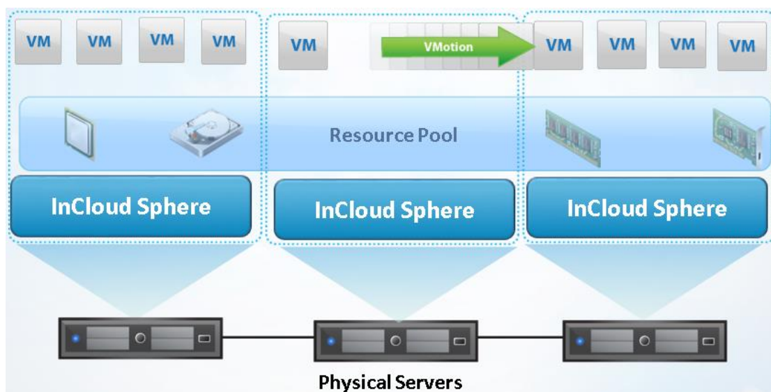
图 4.4.1-1 vMotion 示意图
