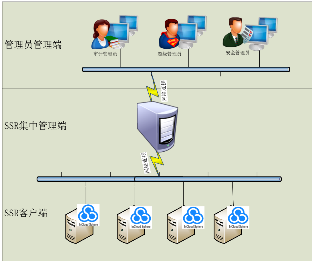
图 6.5.2-1 SSR 工作原理图
