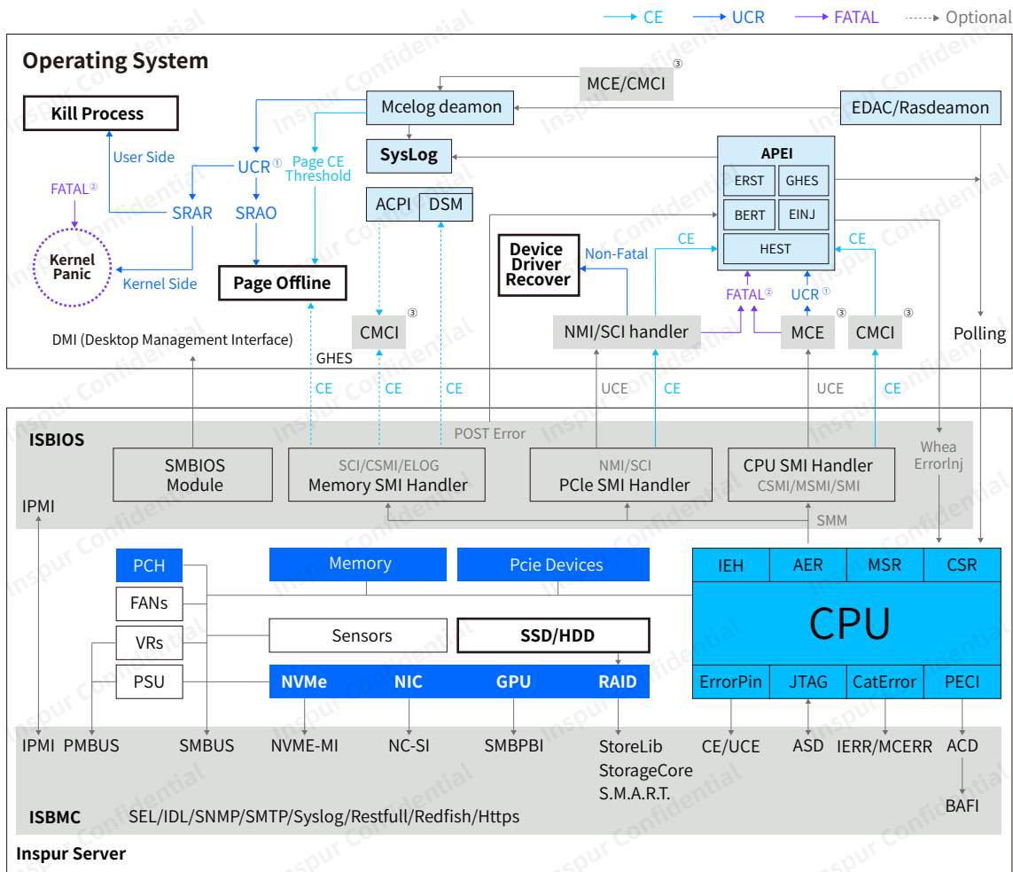
图3-7 服务器故障处理流程
