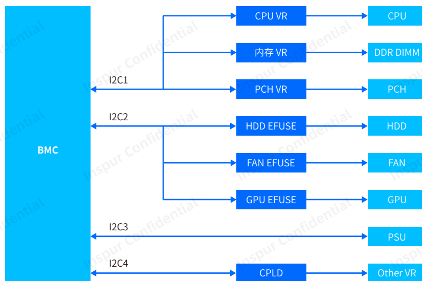
图5-3 常见服务器VR & Efuse错误定位拓扑
